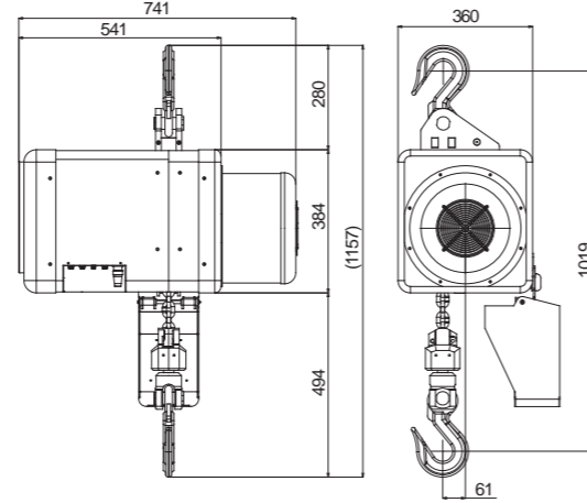
MLH-2000K
