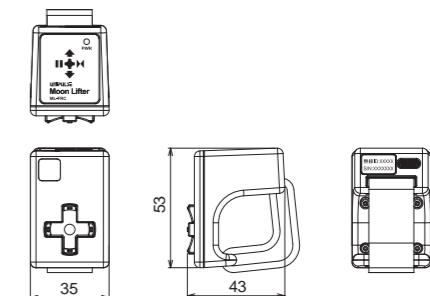
ML-FRC
