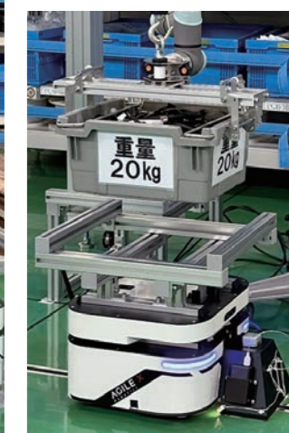
コンテナをAGVに移送
